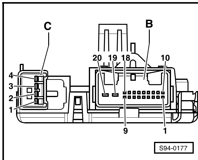
Рис. 1: Штекерный соединитель центрального блока управления электрической бортовой сетью -J519- -В-
